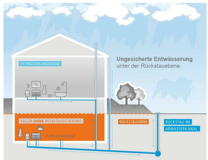
Abbildung: Darstellung einer Hausentwässerung bei Rückstau ohne Rückstausicherung. Grafik: Wasserwerke Zwickau
